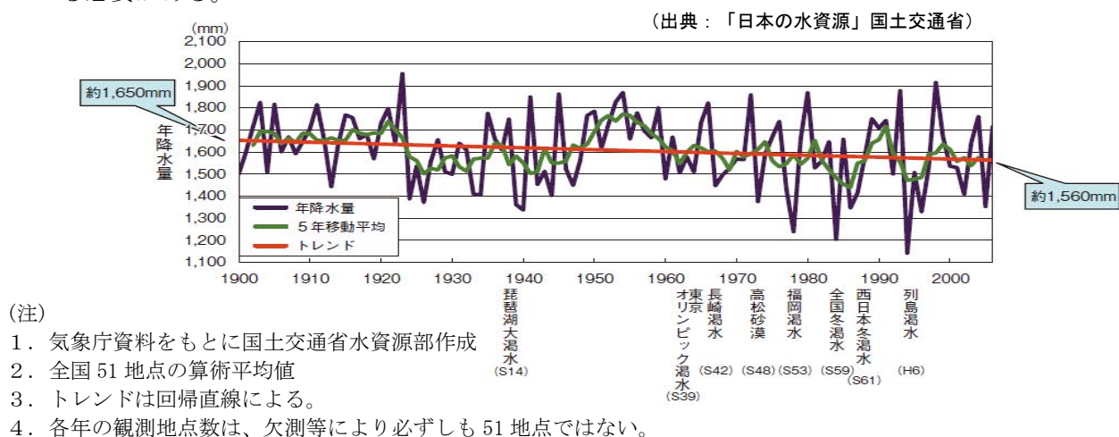
図 2.2.11 日本の年降水量の経年変化
