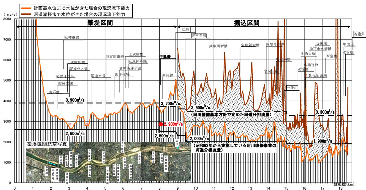
図 2.2.4 現況流下能力
