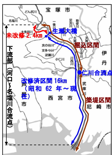
図 2.2.2 河川改修事業の実施範囲
