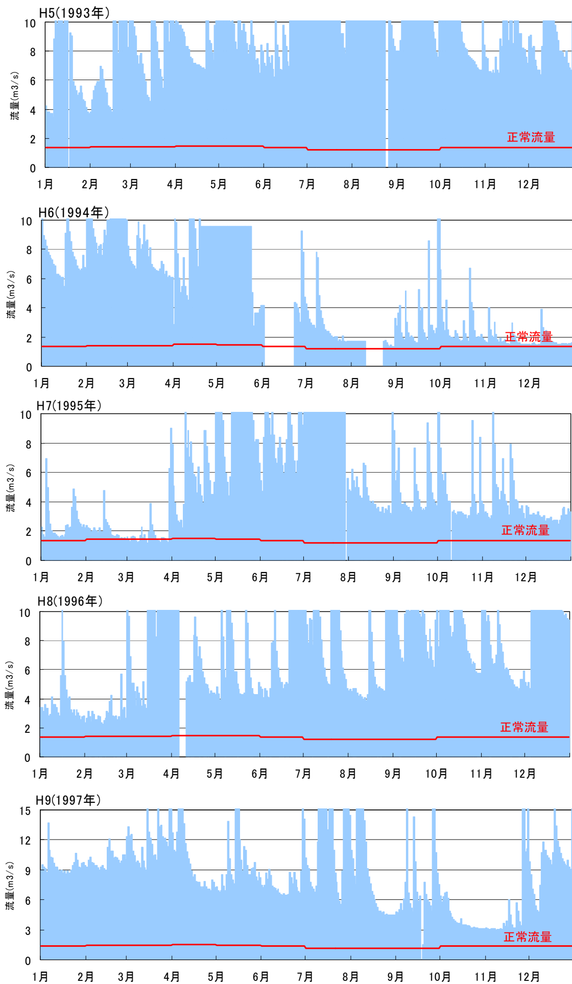
図 5.3(1) 日平均流量図(生瀬橋地点：H5～H9)
