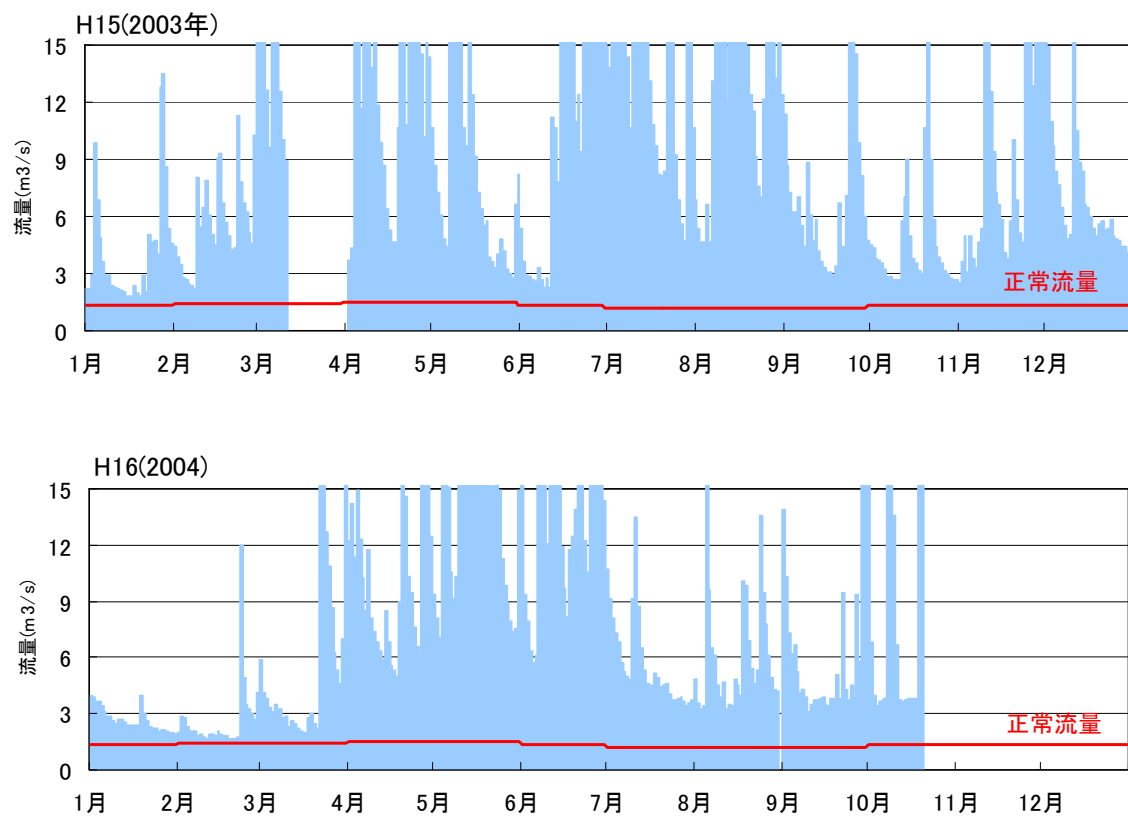
图 5.3 (3) 日平均流量图(生瀬橋地点：H15~H16)
