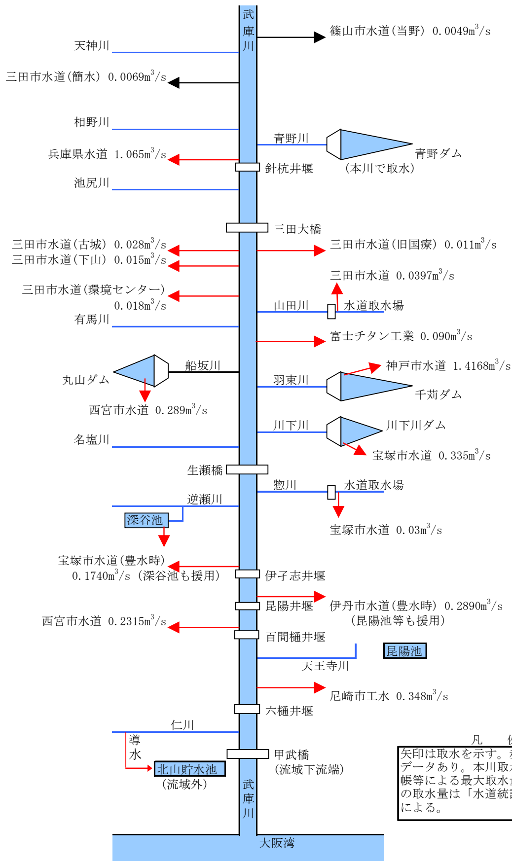
図 1.1 武庫川からの取水模式図（水道用水・工業用水）
